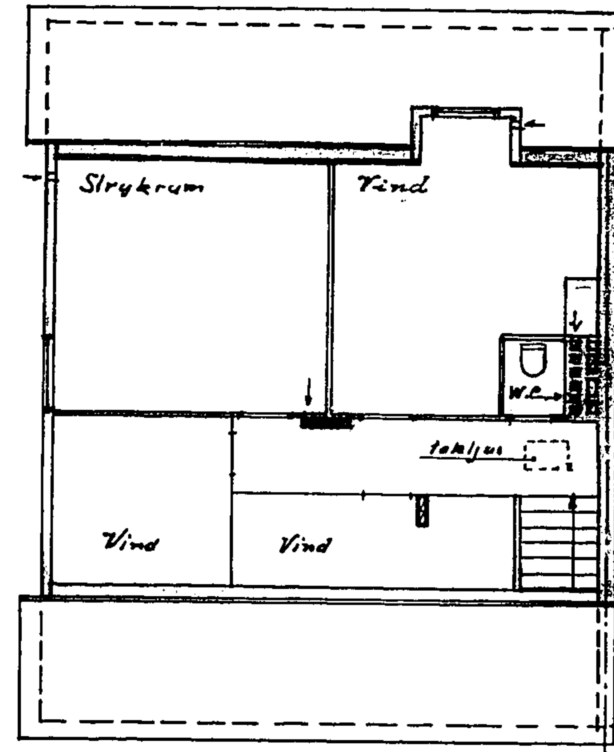
Plan av vinden
