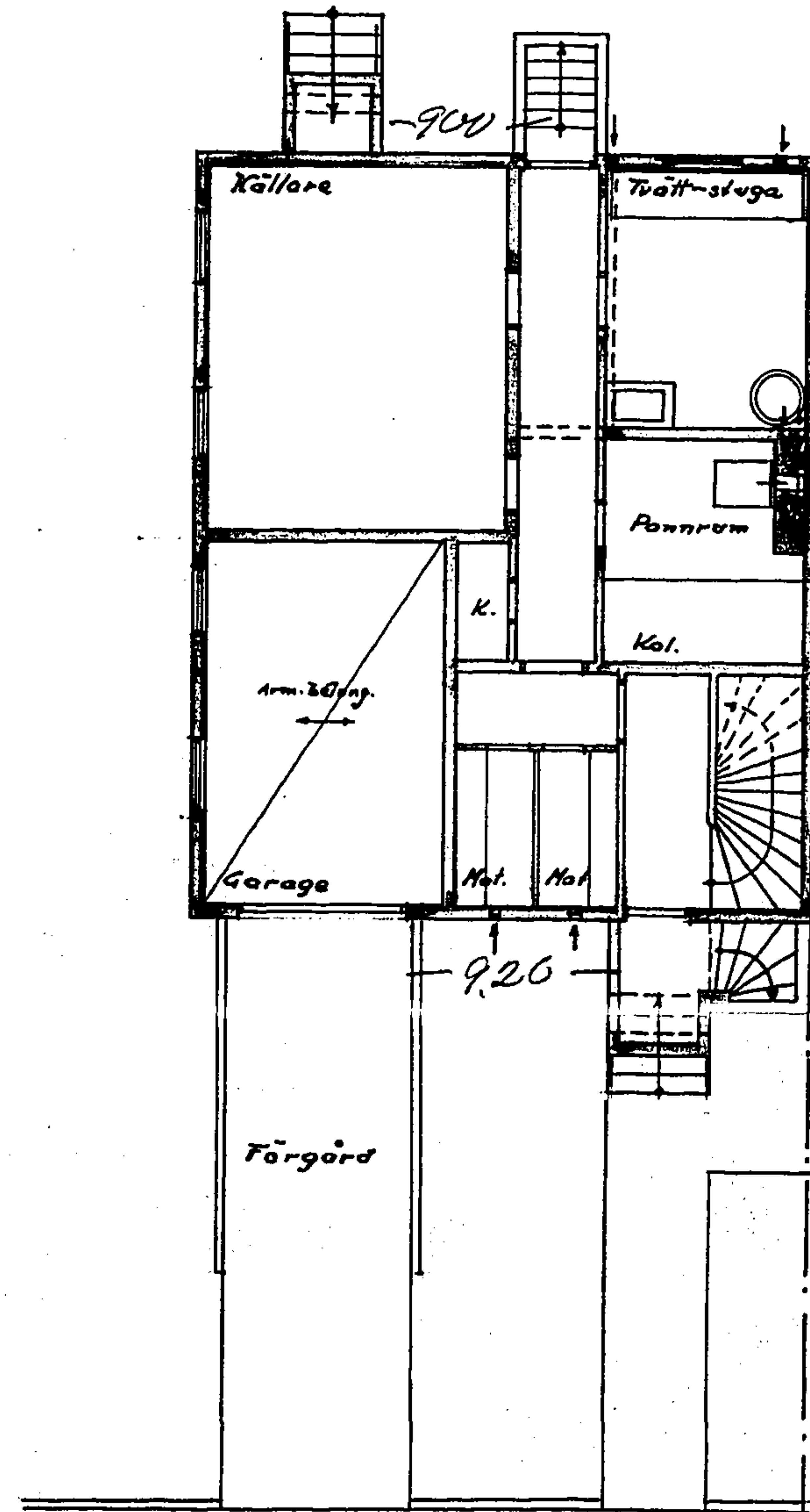
Plan av källaren
